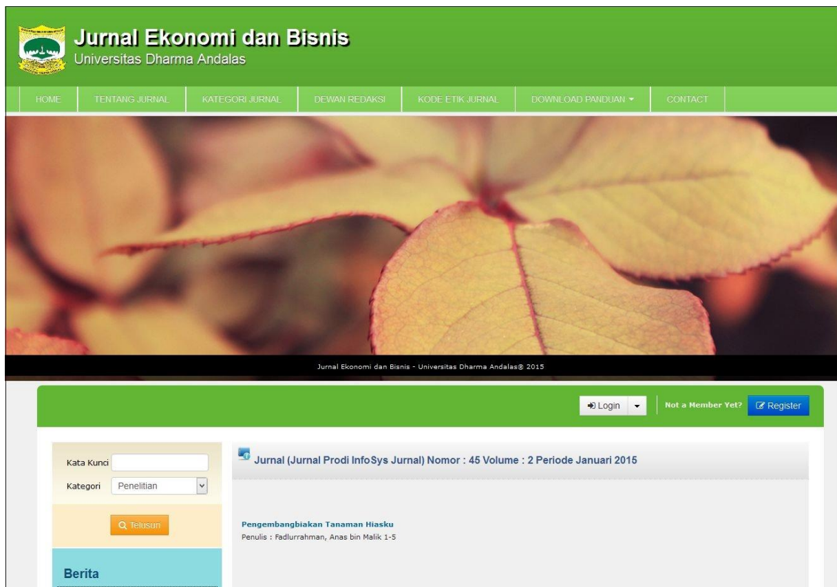
Gambar 1. Halaman Utama
